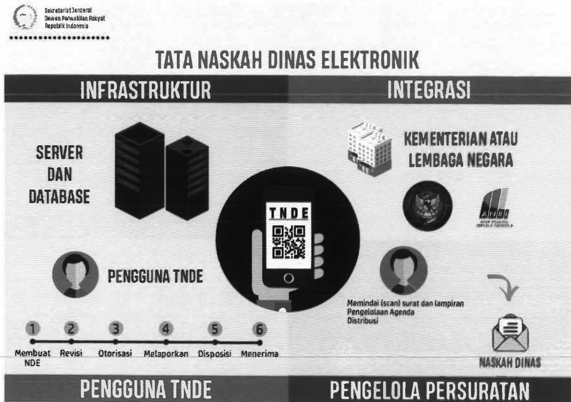
Gambar 1. Arsitektur TNDE
