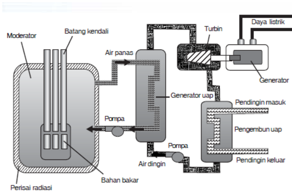
Gambar 1 Komponen Reaktor Nuklir
